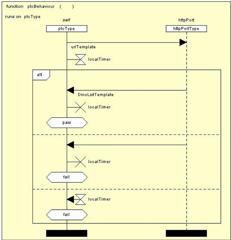
Fig. 4. A GFT Function
